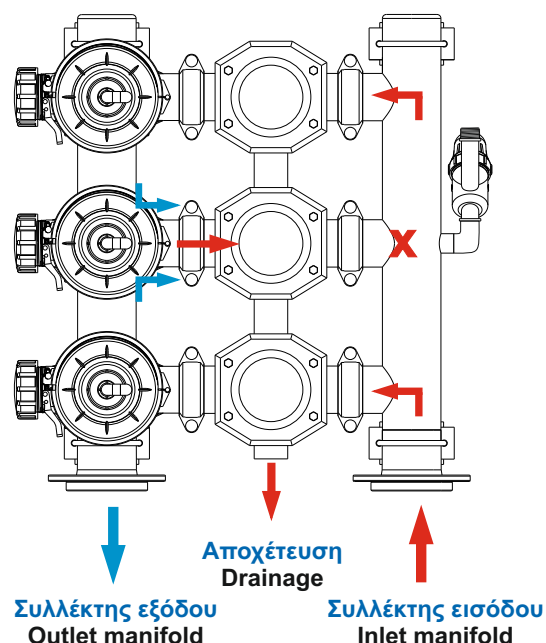
Διαδικασία αυτοκαθαρισμού Self-cleaning procedure
